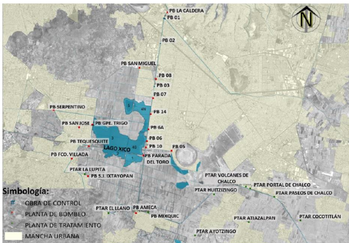
Figura 6 Esquema Infraestructura hidráulica alrededor del Lago Tláhuac - Xico
