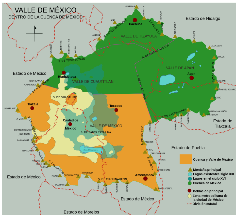
Figura 1. Cuenca de México con los valles que la componen.
